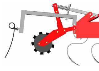
Rouleau + herse peigne flottante
